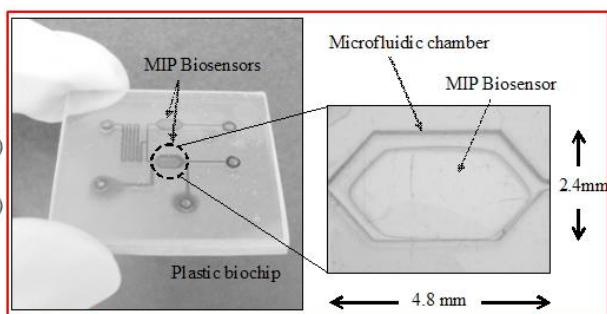
高專一性麻藥感測器及微流體晶片
